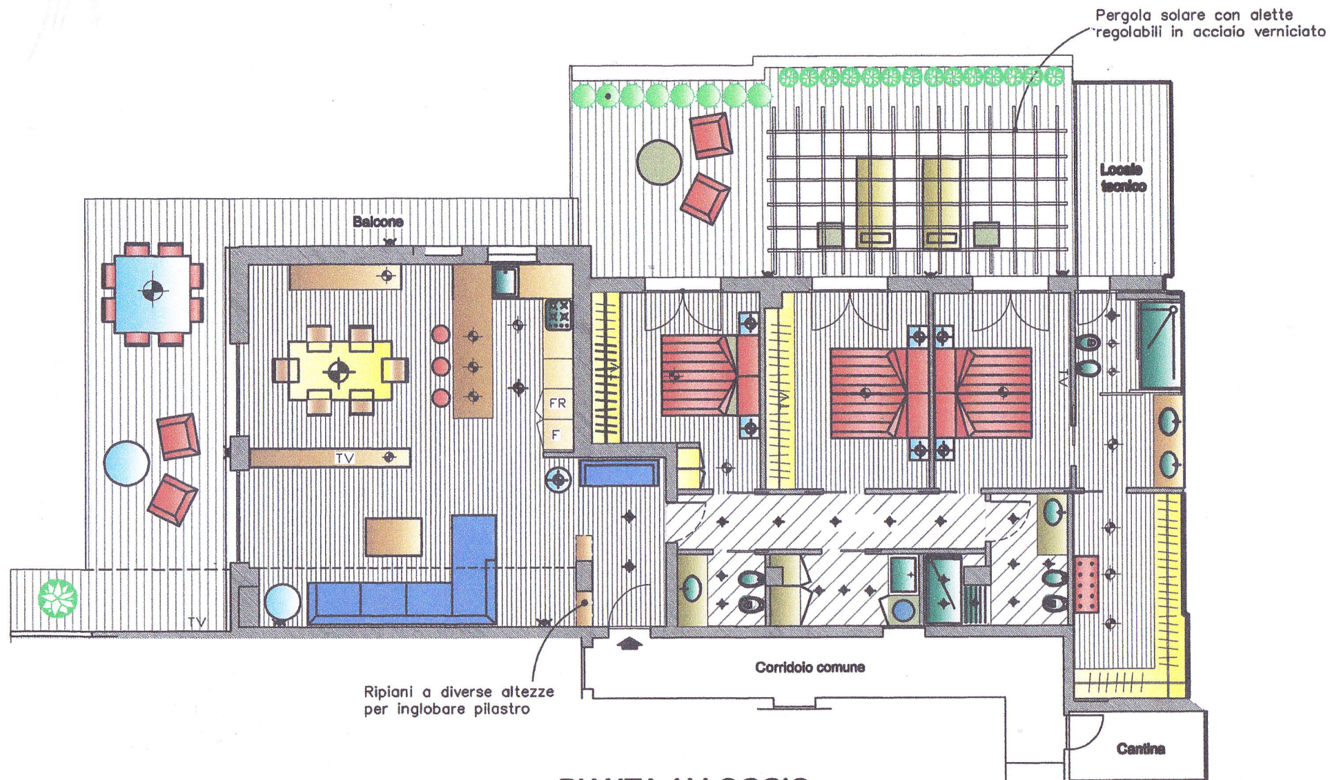
PIANTA ALLOGGIO Arredamento
